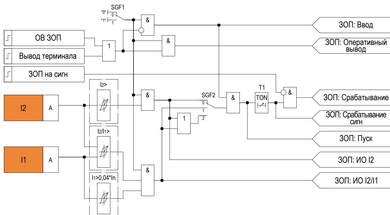
Рисунок 2.28 – Функциональная схема логики 3ОП
